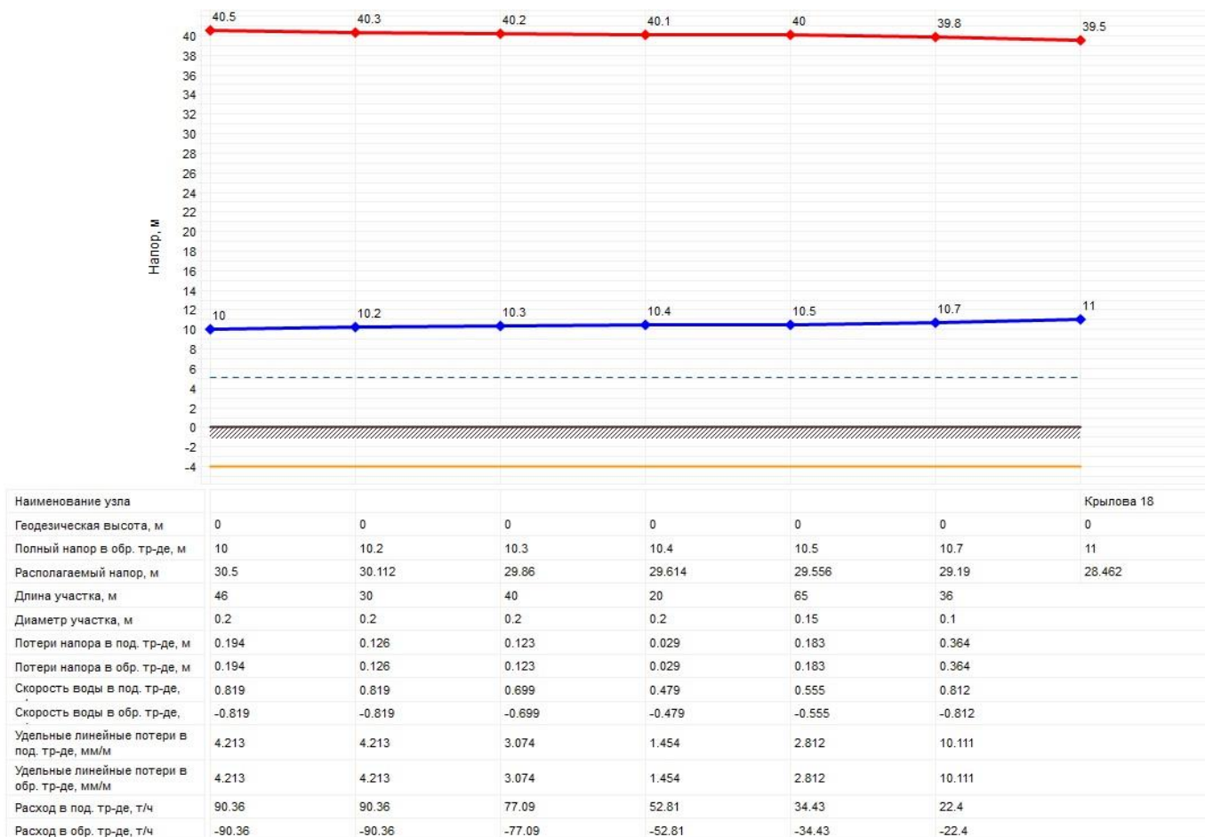
Рисунок 2.33 – Пьезометрический график от источника теплоснабжения (Котельной №2 с. Кичигино) до самого удаленного потребителя
