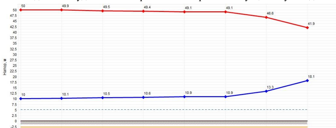
Рисунок 2.44 – Пьезометрический график от Котельной п. Нагорный до самого удаленного потребителя в аварийной ситуации по ул. Садовая
