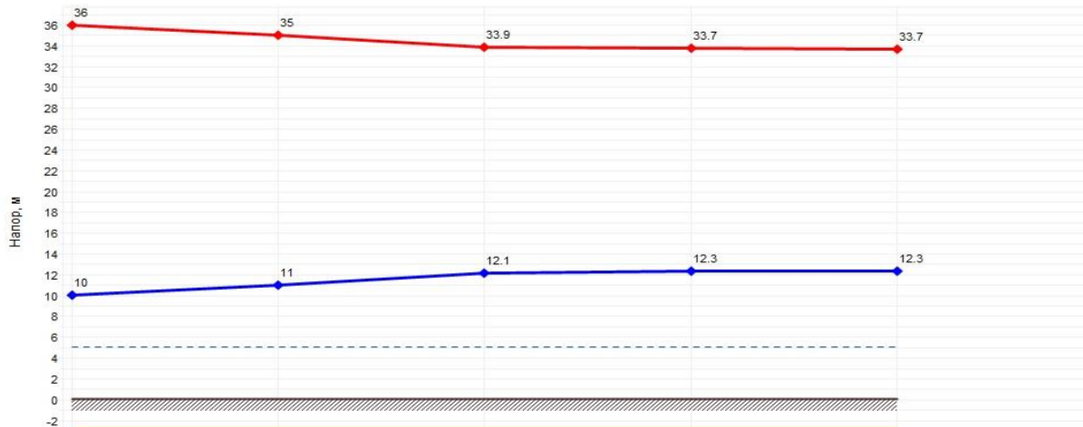
Рисунок 2.35 – Пьезометрический график от источника теплоснабжения (Котельной п. Нагорный) до самого удаленного потребителя – детского сада
