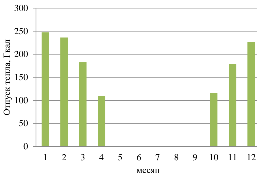
Рисунок 1.9 Оптимальный температурный график отпуски тепловой энергии для Котельная п. Синий Бор с температурным режимом 90-70 °С
