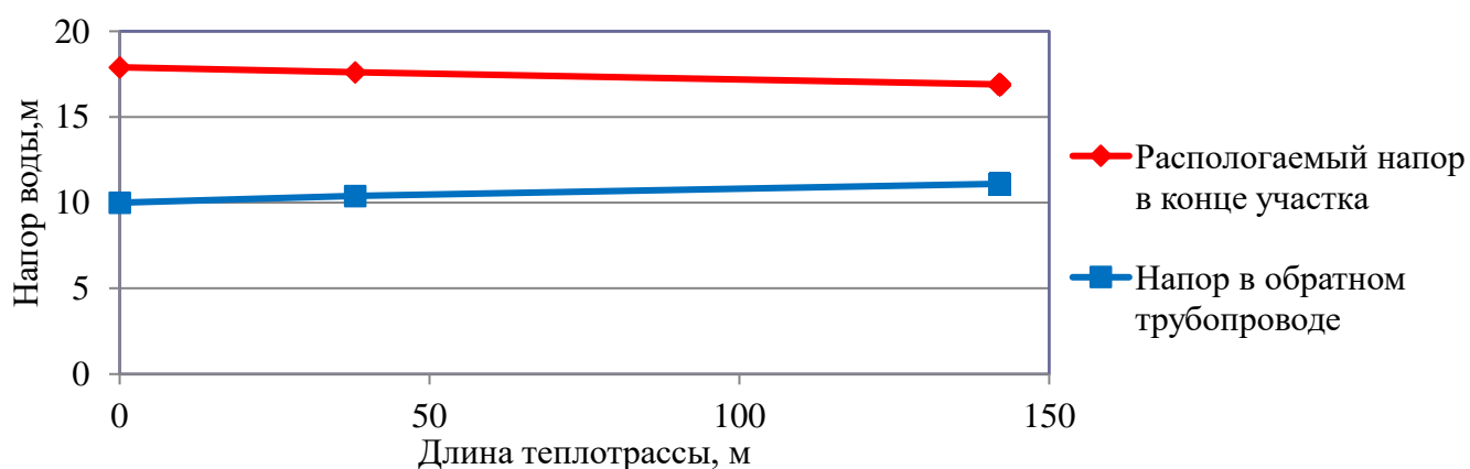
Рисунок 2.7 – Пьезометрический график тепловой сети Котельной №1 с. Кичигино
